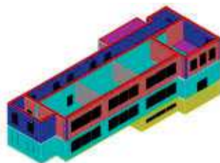
Progetto di interventi per miglioramento strutturale edificio scolastico scuola elementare “Giovanni XXIII”
