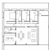
Pianta del Piano Terra
