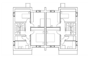
Pianta del Piano Primo
